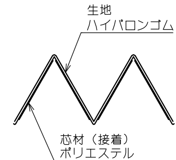
ジャバラ詳細図
